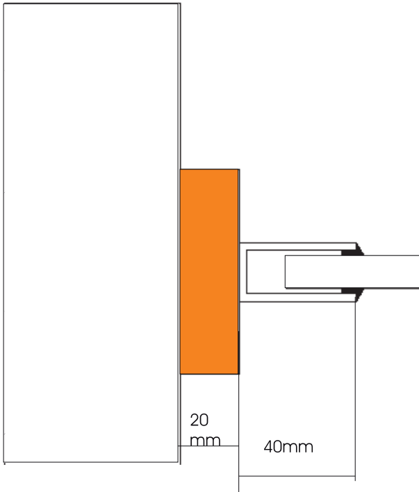
Deckenanschluß mit zusätzlichem Holzprofil
